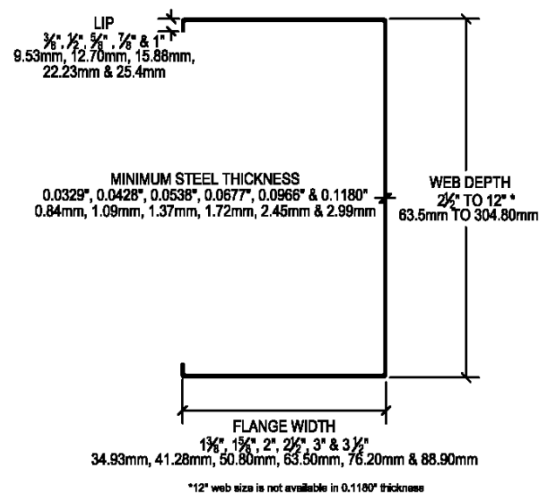
STRUCTURAL STUD
